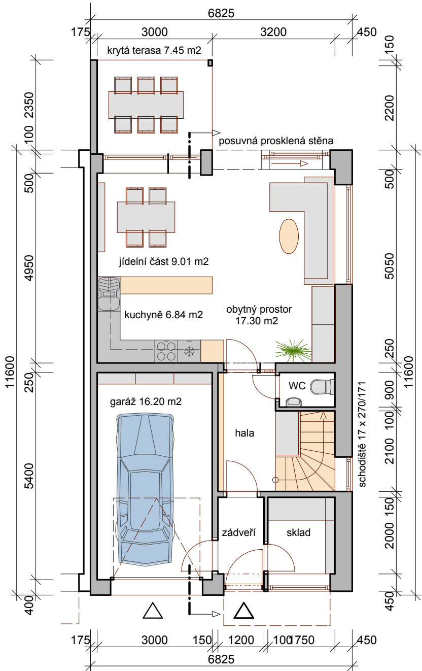
Půdorys přízemí
